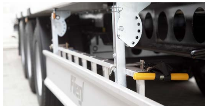
Hinter dem klappbaren Unterfahrschutz sind Halterungen für Zubehör wie Leiter, Besen und Schaufel angebracht.
