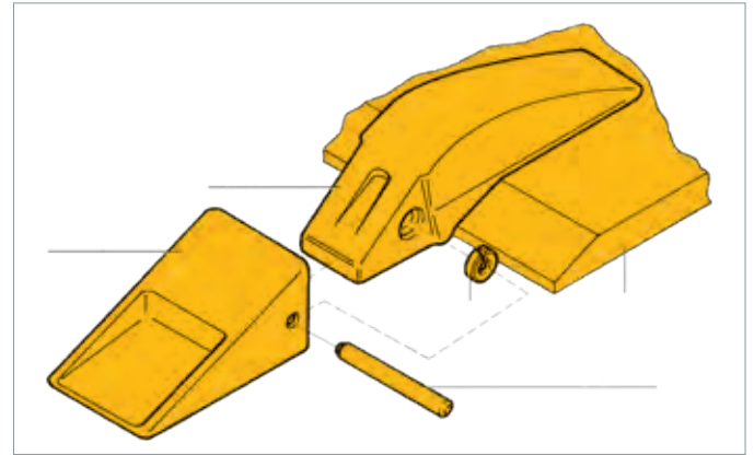
Zweiteilige Zähne mit leicht auswechselbarer Zahnspitze
