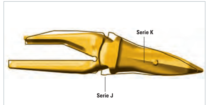
Profilvergleich J-K-System
